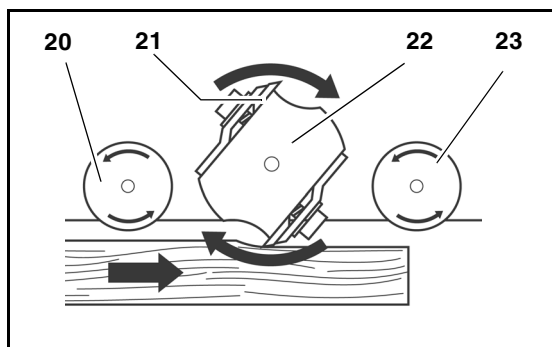
Planhyvelns princip
